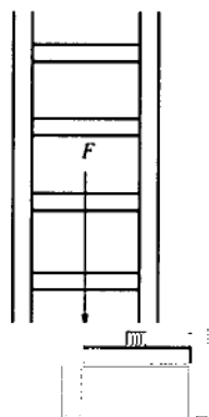
图 B.7 侧面挠度试验布置图
